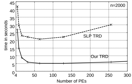
(a) n = 2000 の場合
