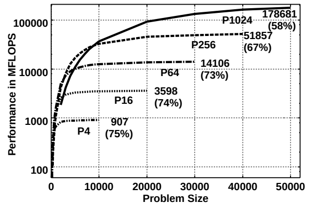
図 2 三重対角化ルーチンの性能
